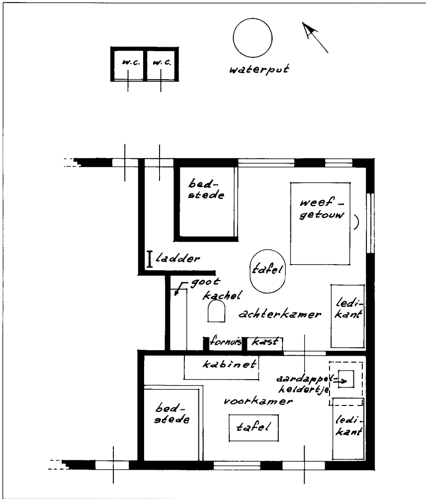
Plattegrond van de weverswoning van Jaonneke Janssens, Hasselstraat 231, Tilburg (ca. 1900). Reconstructie Ton Wagemakers (tekening John Goeyjers, gemeente-archief 1985)
